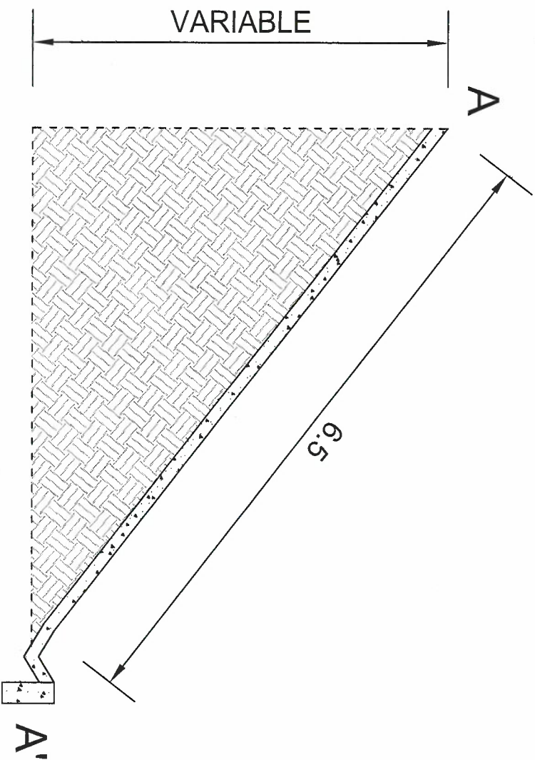
3 CORTE A - A' Scale: 1:50
