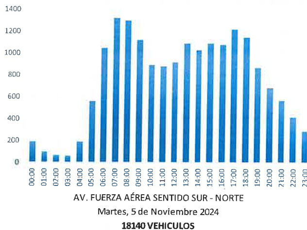
GRAFICA 13. Volumen vehicular durante 24 hrs. Punto seccional no.2
