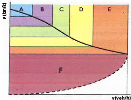
Representación de los niveles de servicio en el diagrama de volumen y velocidad
