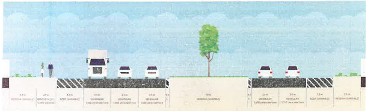
IMG. 12. Sección propuesta por PDU en Carretera Chihuahua a Aldama
