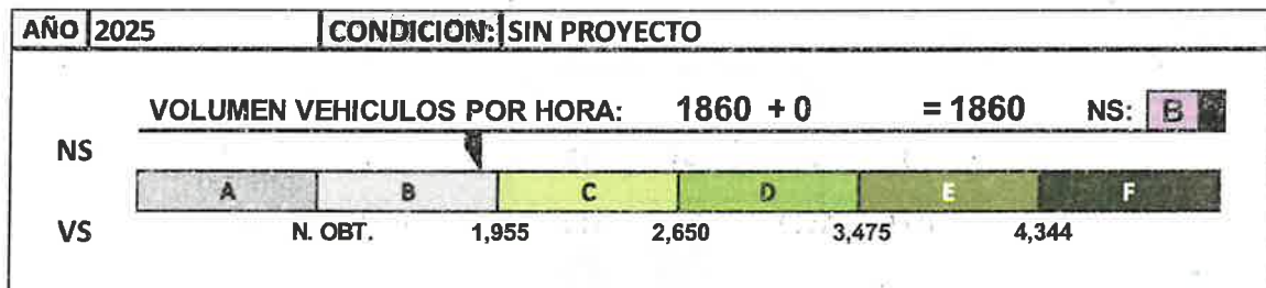
GRAFICA 29. Volúmenes de capacidad para cada nivel de servicio
