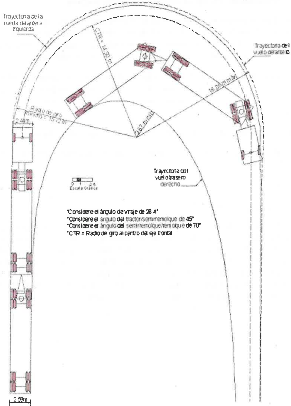
IMG. 27. Dimensiones de giro del vehículo TSR
