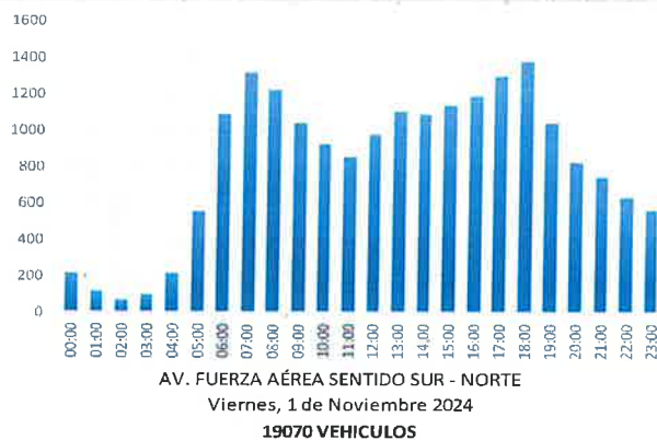
GRAFICA 9. Volumen vehicular durante 24 hrs. Punto seccional no.2
