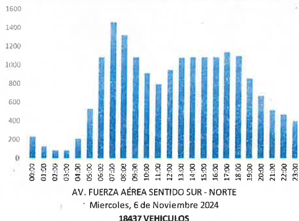
GRAFICA 14. Volumen vehicular durante 24 hrs. Punto seccional no.2
