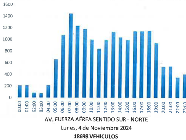
GRAFICA 12. Volumen vehicular durante 24 hrs. Punto seccional no.2
