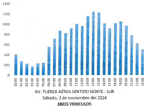
GRAFICA 3: Volumen vehicular durante 24 hrs. Punto seccional No.1
