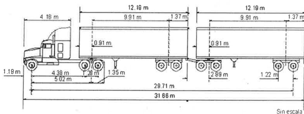
IMG. 26. Dimensiones generales de vehículo TSR.
