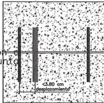
Vista en planta Translación horizontal
