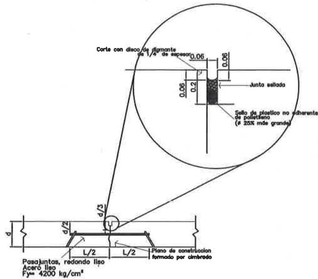
Corte y sellado de junta de construcción transversal con barra amarre
