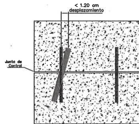
Vista en planta Esviajamiento horizontal
