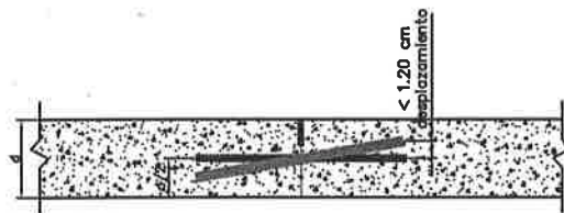
Vista en corte. Esviajamiento vertical
