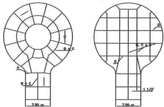
PLANTA DE LOCALIZACION DE JUNTAS PARA CUL-DE-SAC
