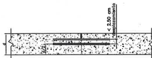
Vista en corte Translación vertical
