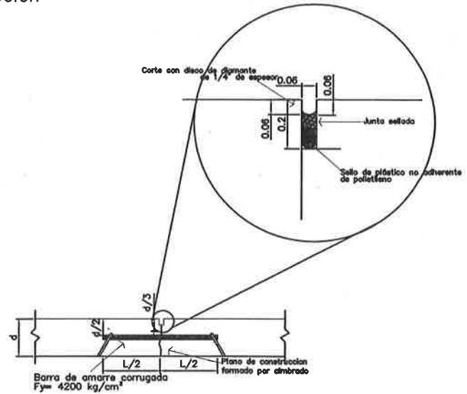
Corte y sellado de junta de construcción longitudinal con barra amarre
