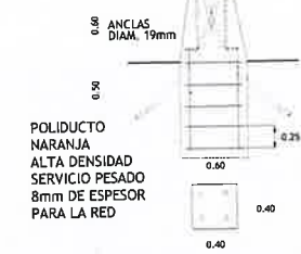
DETALLE DE ZANJAS
