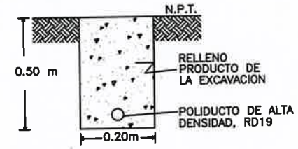
DETALLE DE ZANJAS
