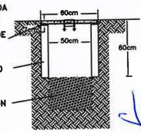
DETALLE DE REGISTRO
