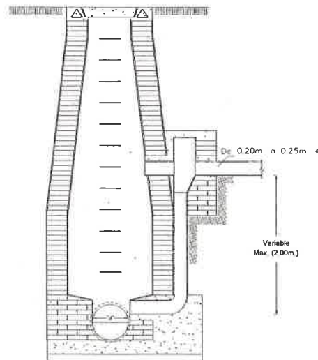
TRAMO CABECERO O DE ARRANQUE DEL SISTEMA
