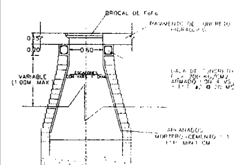
06 Detalle de Pozo de Visita
