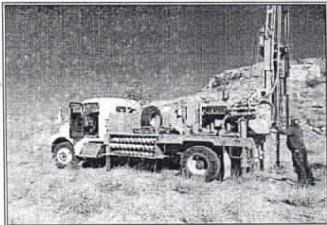
PERFORADORA COLOCADA EN EL PUNTO DEL SONDEO SP-3
