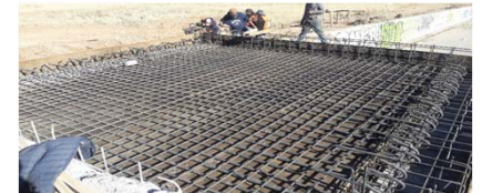
APROCHE EN ESTRIBO IZQUIERDO
