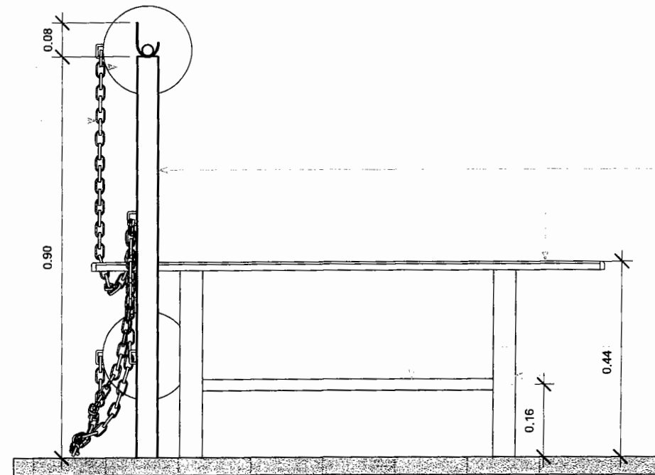
4 ELEVACIÓN 03 1 : 10
