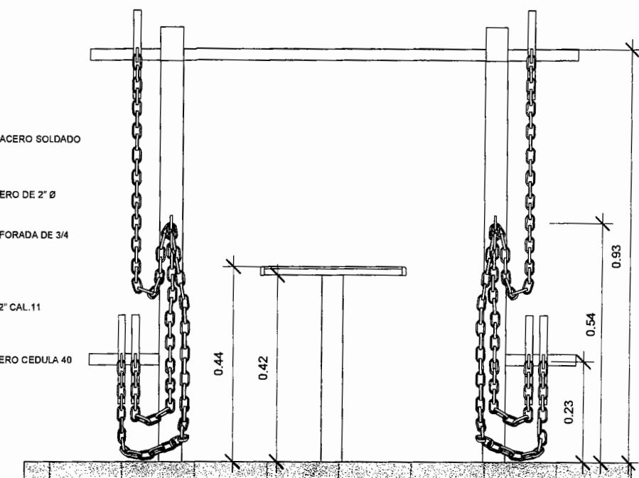
3 ELEVACIÓN 02 1 : 10
