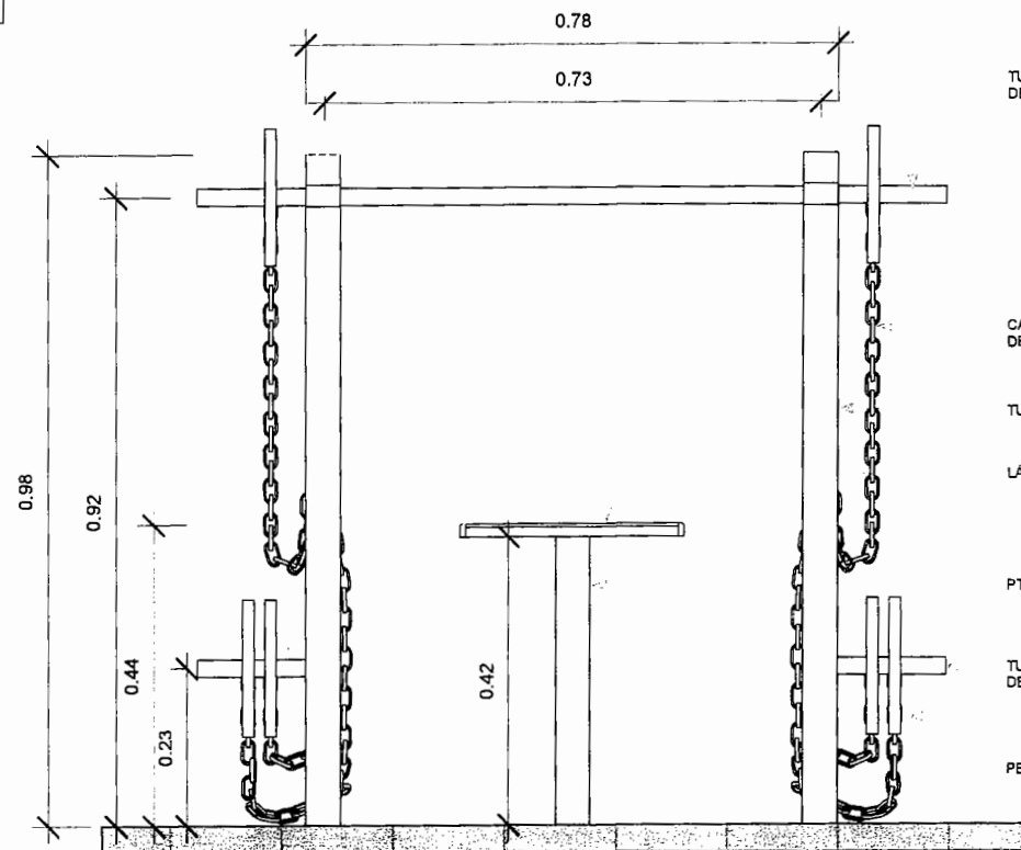
2 ELEVACIÓN 01 1 : 10
