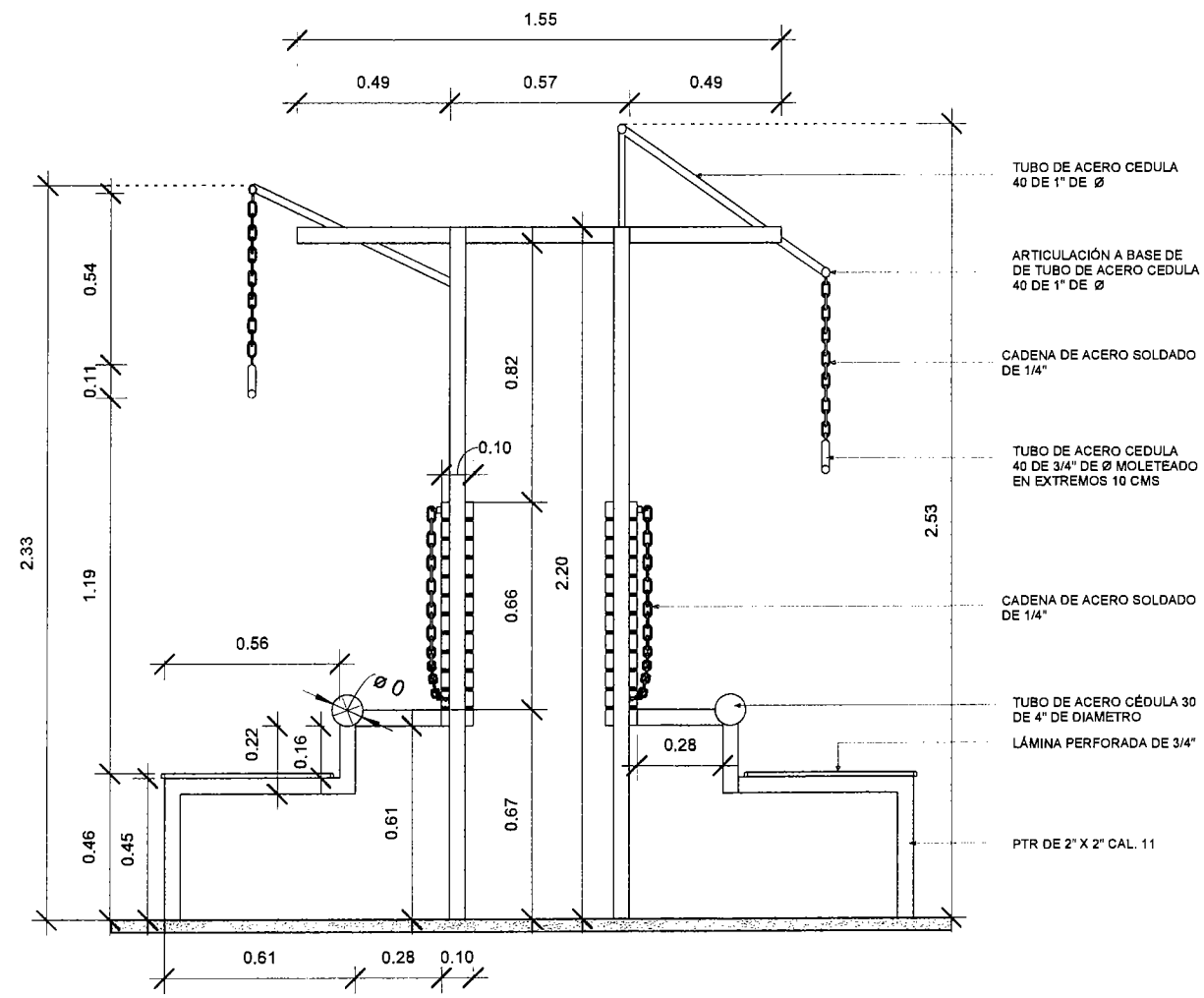
3 ELEVACIÓN 02 1 : 20
