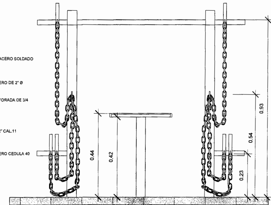
3 ELEVACIÓN 02 1 : 10
