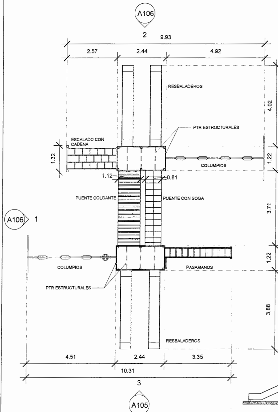
1 JUEGOS INFANTILES 1 : 100
