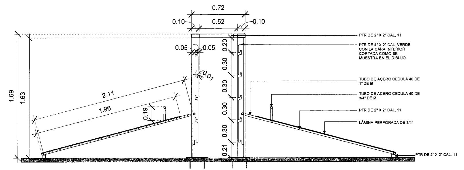
4 SECCIÓN 01 1 : 25
