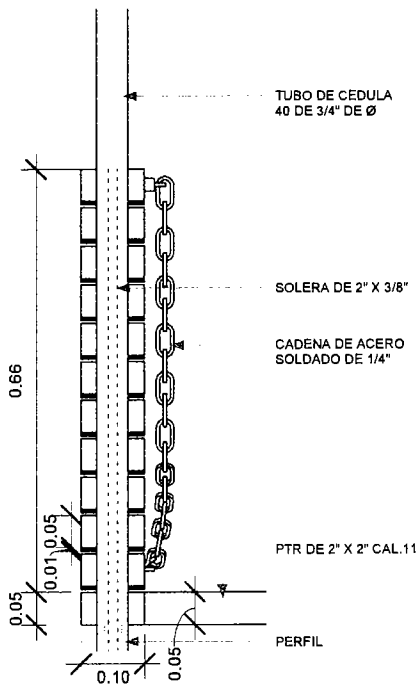
2 DETALLE DE PESAS 1 : 10
