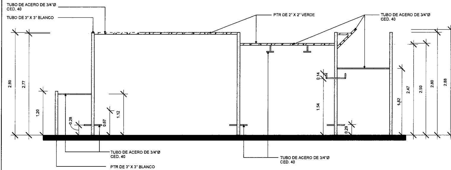
3 Elevación 3 1 : 50
