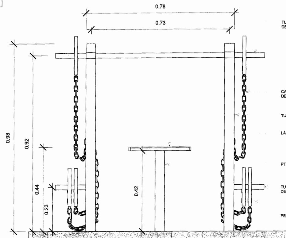
2 ELEVACIÓN 01 1 : 10
