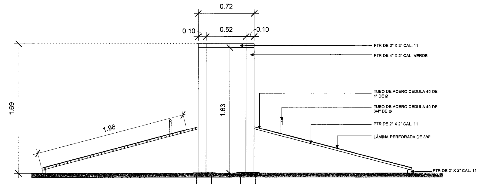
2 ELEVACIÓN 01 1 : 25
