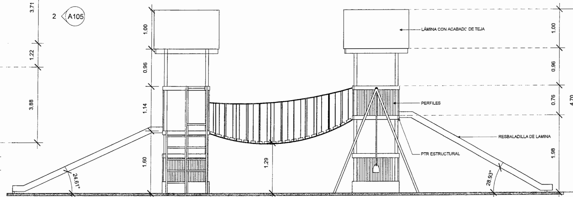
2 ELEVACIÓN 01 1 : 50
