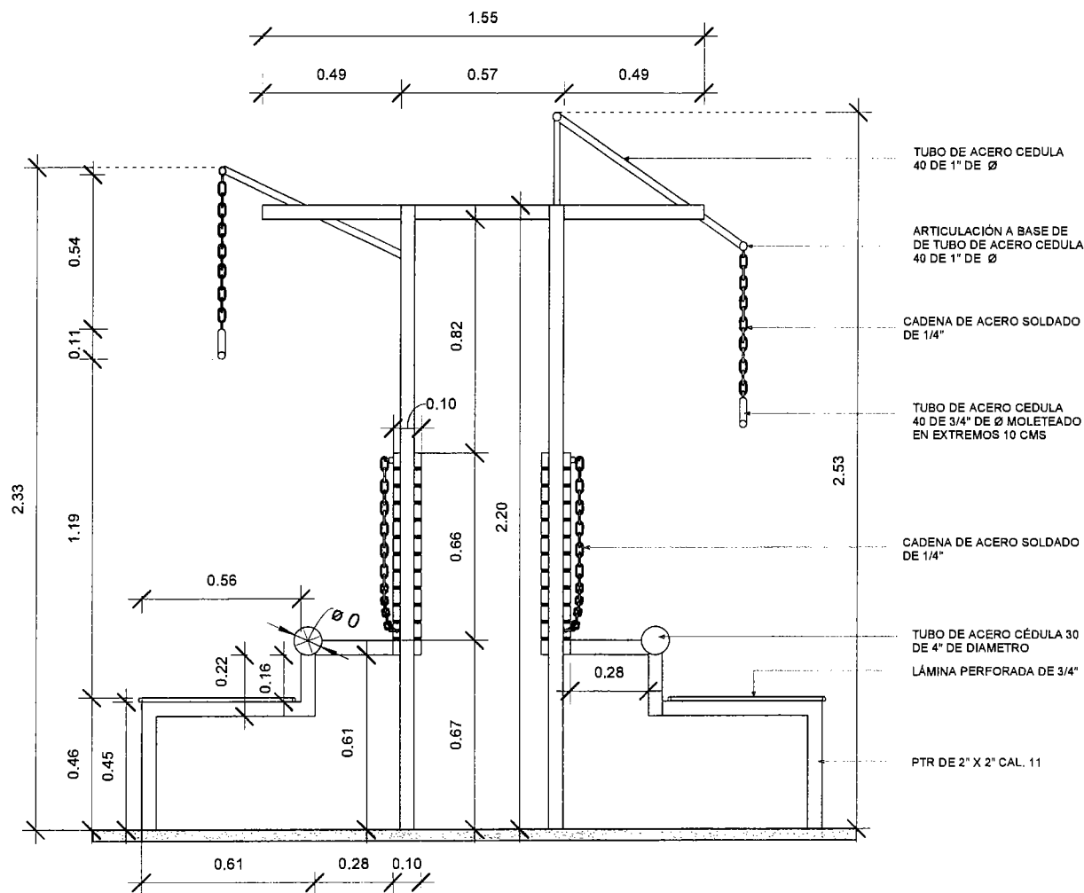
3 ELEVACIÓN 02
