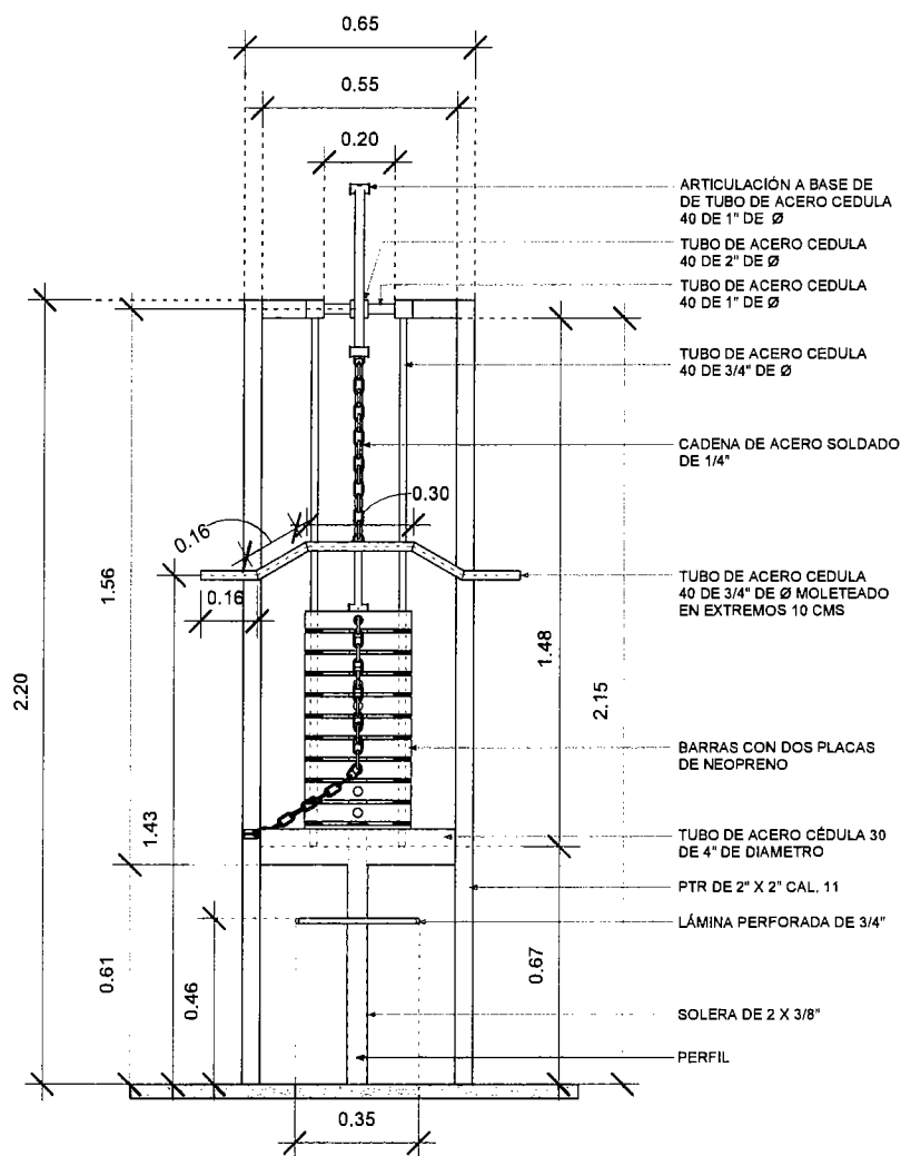
2 ELEVACIÓN 01
