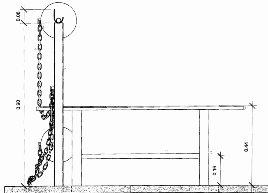
4 ELEVACIÓN 03 1 : 10
