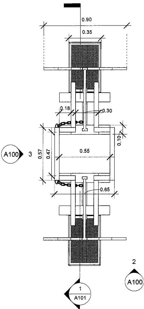
1 PLANTA APARATO 1 : 20
