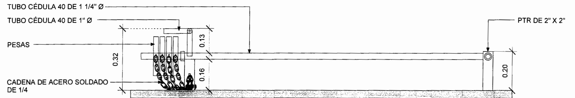
2 Alzado 01 1 : 10
