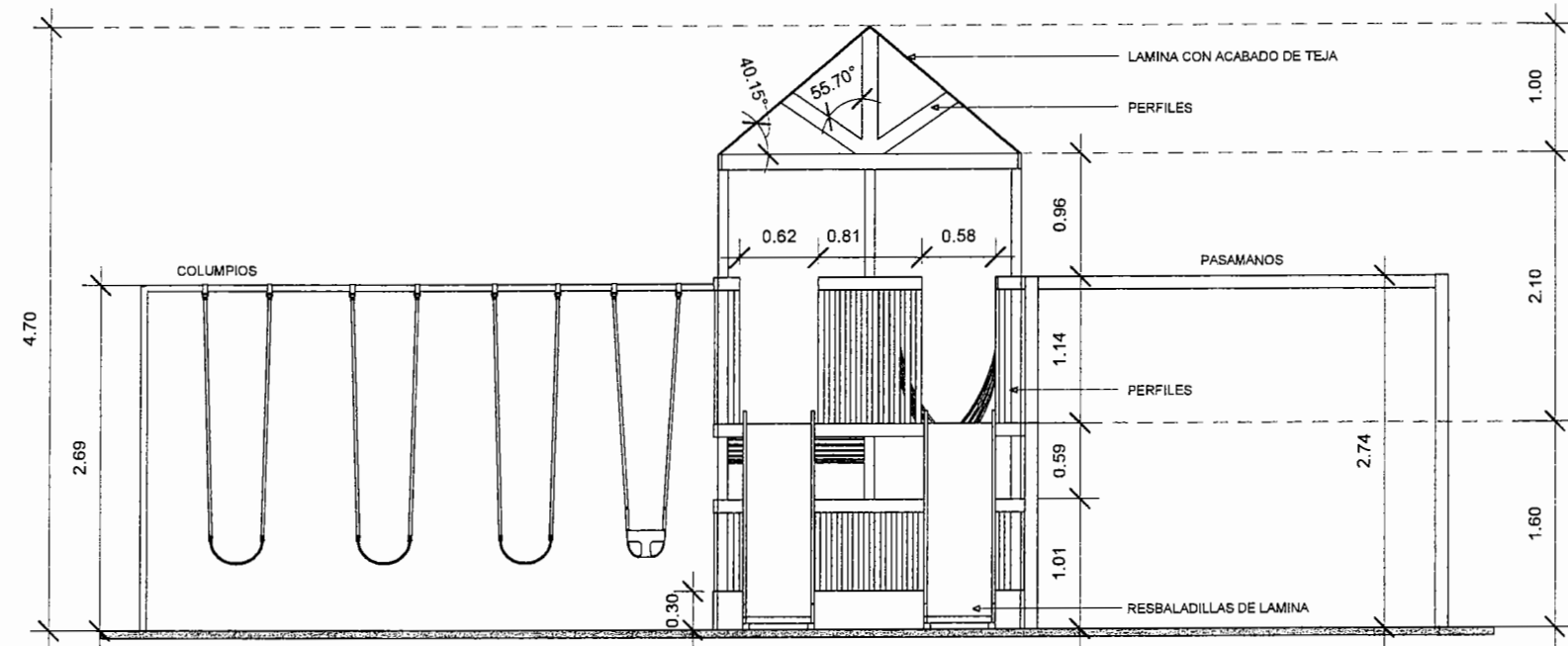
3 ELEVACIÓN 02 1 : 50
