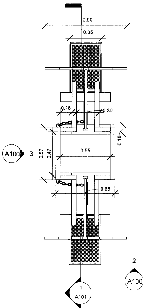
1 PLANTA APARATO
