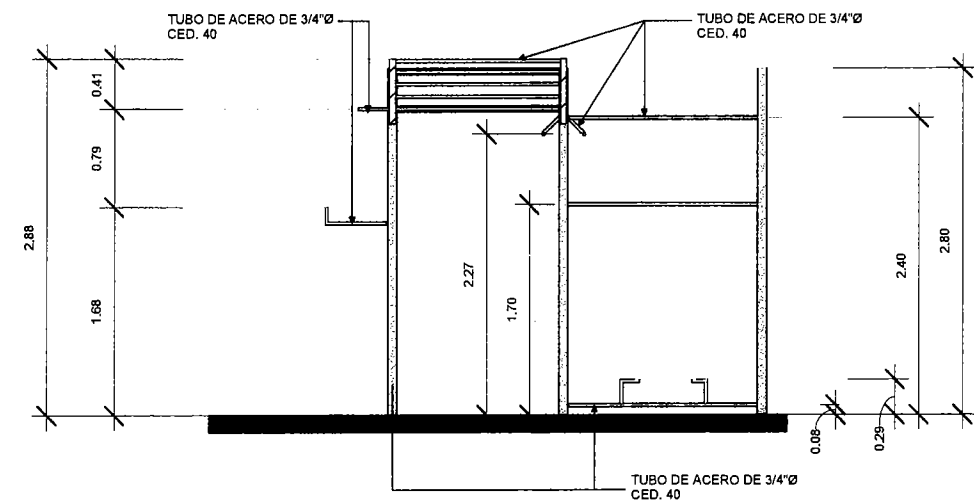
2 Elevación 2 1 : 50
