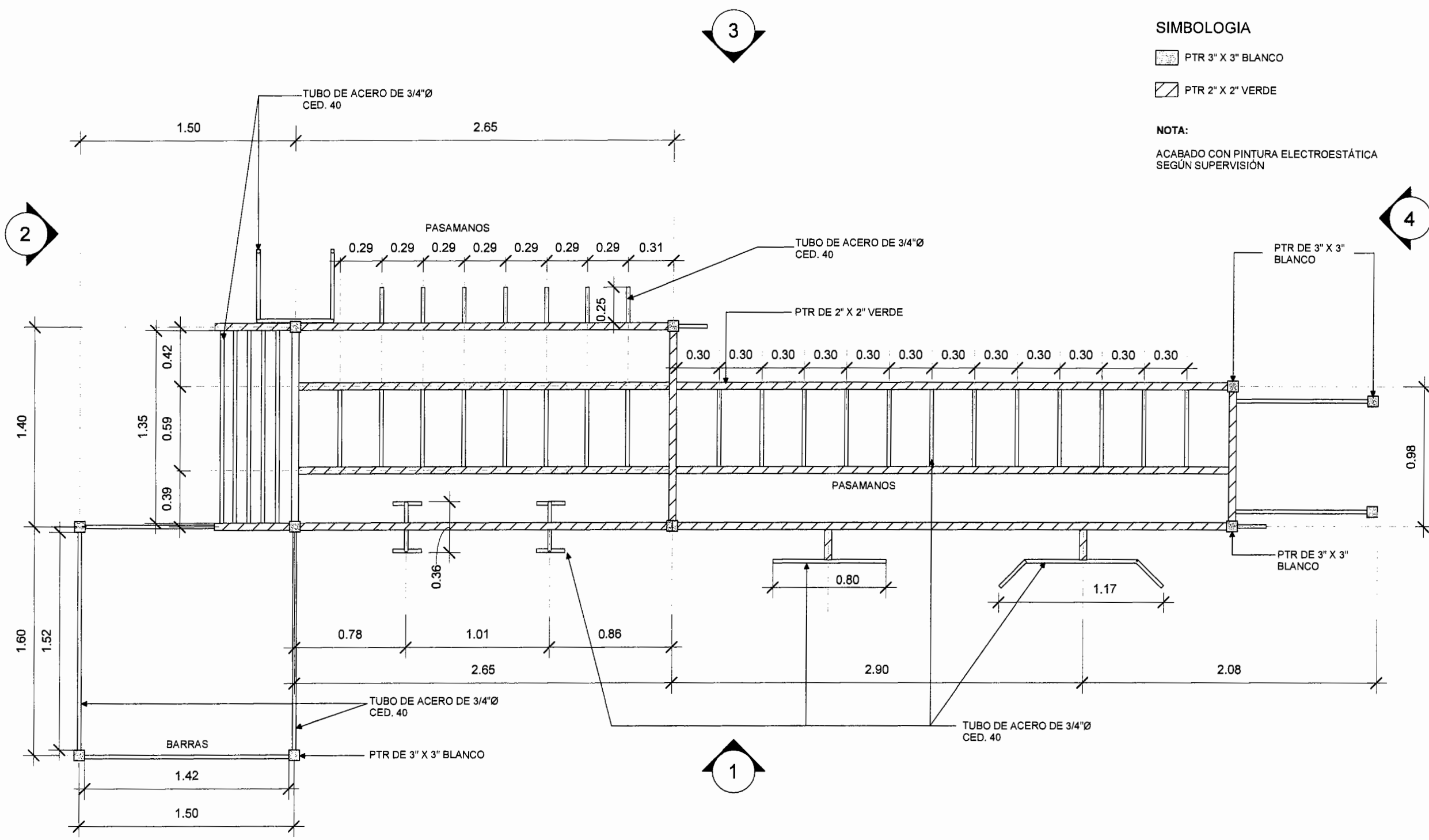
1 Planta Aparato Ejercicios 1 : 25
