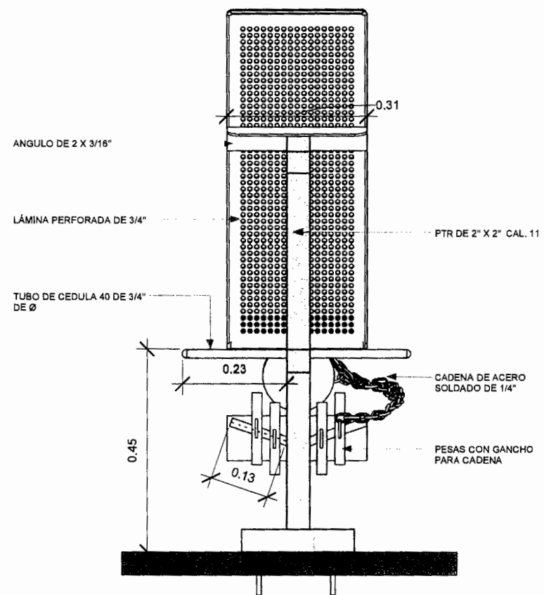
1 ELEVACIÓN 03 1 : 10
