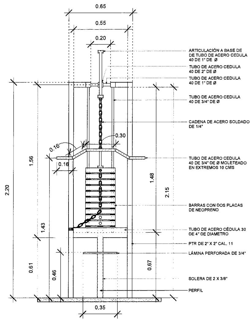
2 ELEVACIÓN 01 1 : 20
