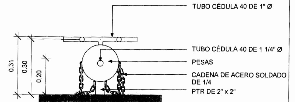
4 Alzado 03 1 : 10
