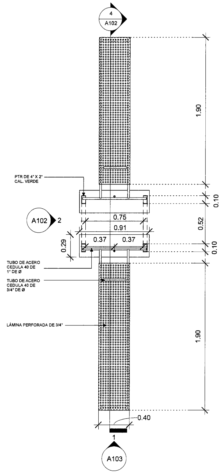
1 APARATO ABDOMINALES 1 : 25
