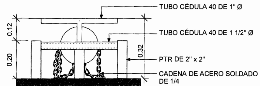
3 Alzado 02 1 : 10
