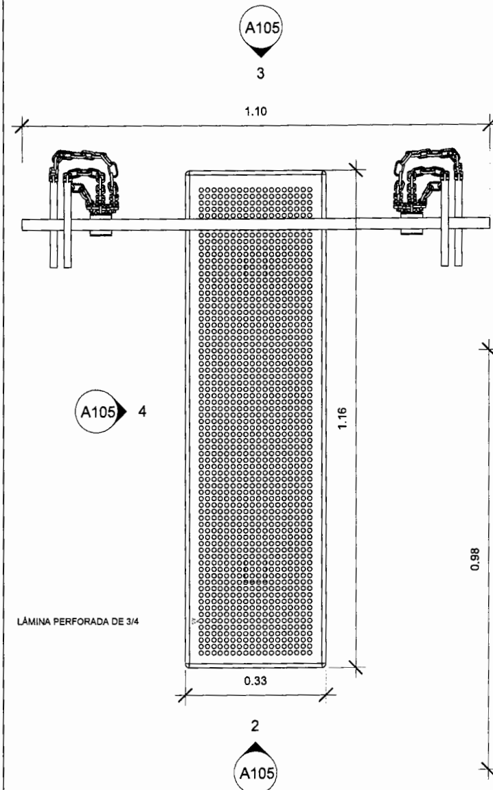
1 APARATO PARA PECHO 1 : 10
