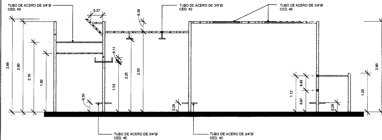
1 Elevación 1 1 : 50
