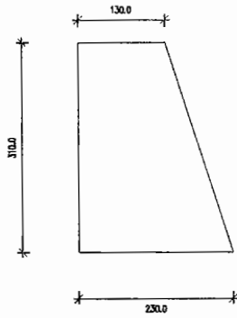
ESTRIBO 2
