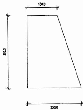
ESTRIBO 1
