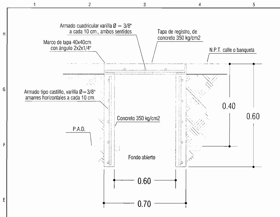
02 DETALLE DE REGISTRO S/E Detalle de registro para sistema de alumbrado público.
