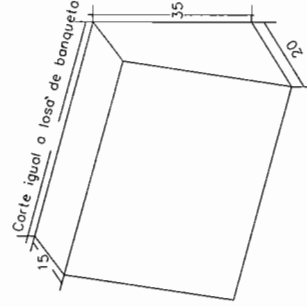
GUARNICION DE CONCRETO
