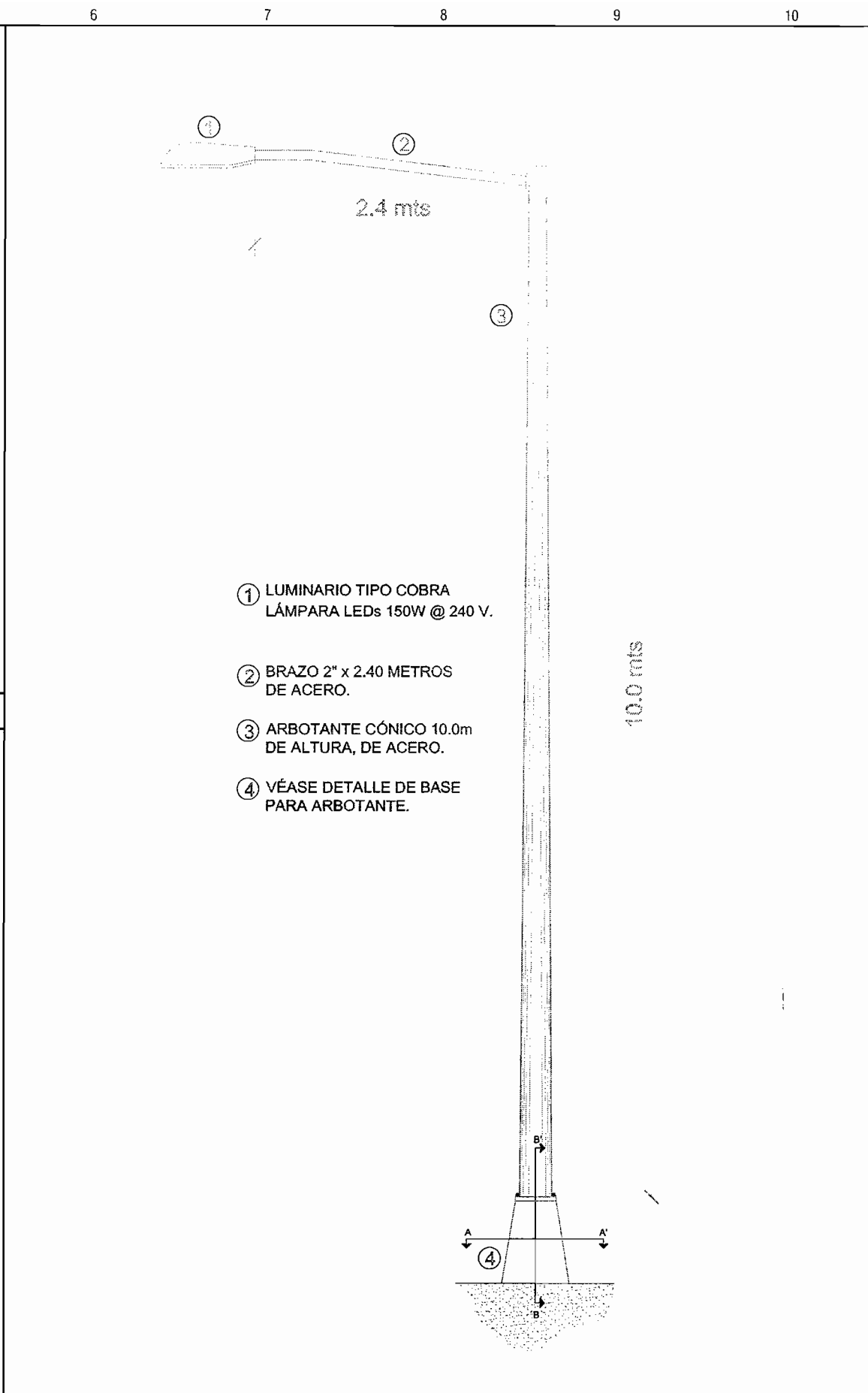
01 DETALLE DE ARBOTANTE 1:40 Detalle de arbotante de alumbrado.
