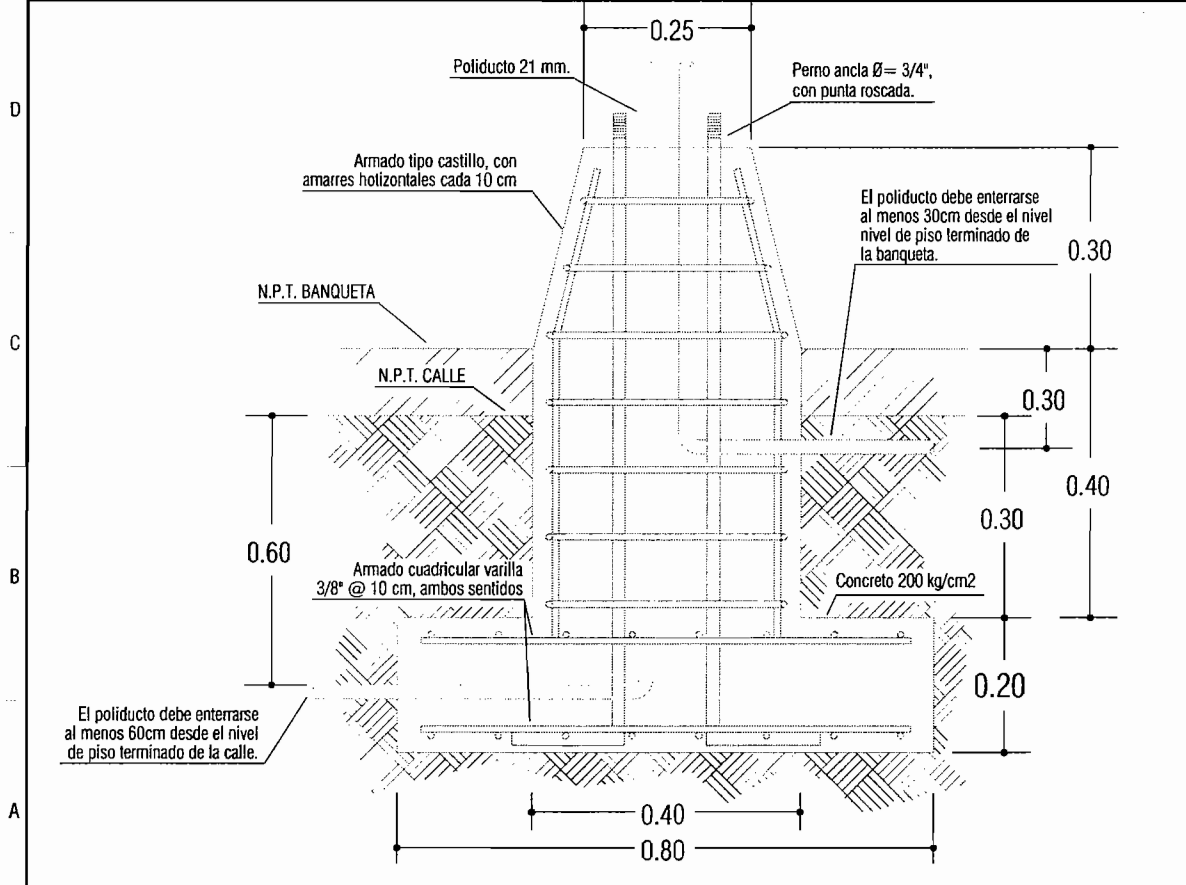
03 DETALLE DE BASE DE ARBOTANTE S/E Detalle para base de arbotante de alumbrado público.
