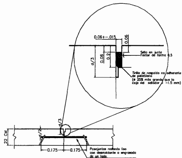
Corte y sellado de junta de contraccion transversal con pasajuntas
