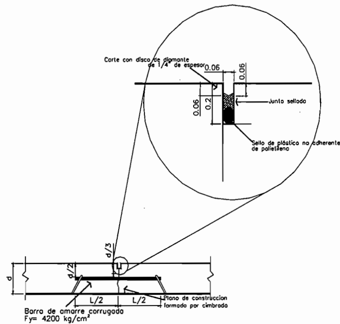
Corte y sellado de junta de construcción longitudinal con barra amarre
