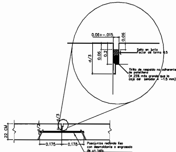
Corte y sellado de junta de contracción transversal con pasajuntas
