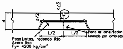
Corte y sellado de junta de construcción transversal con pasajuntas
