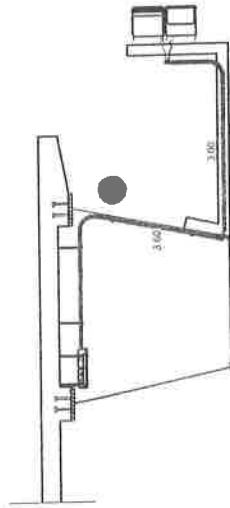
Alimentador de interconexion a luminario lateral tipo (A).
