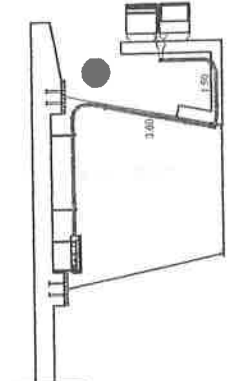
Alimentador de interconexion a luminario lateral tipo (B).
