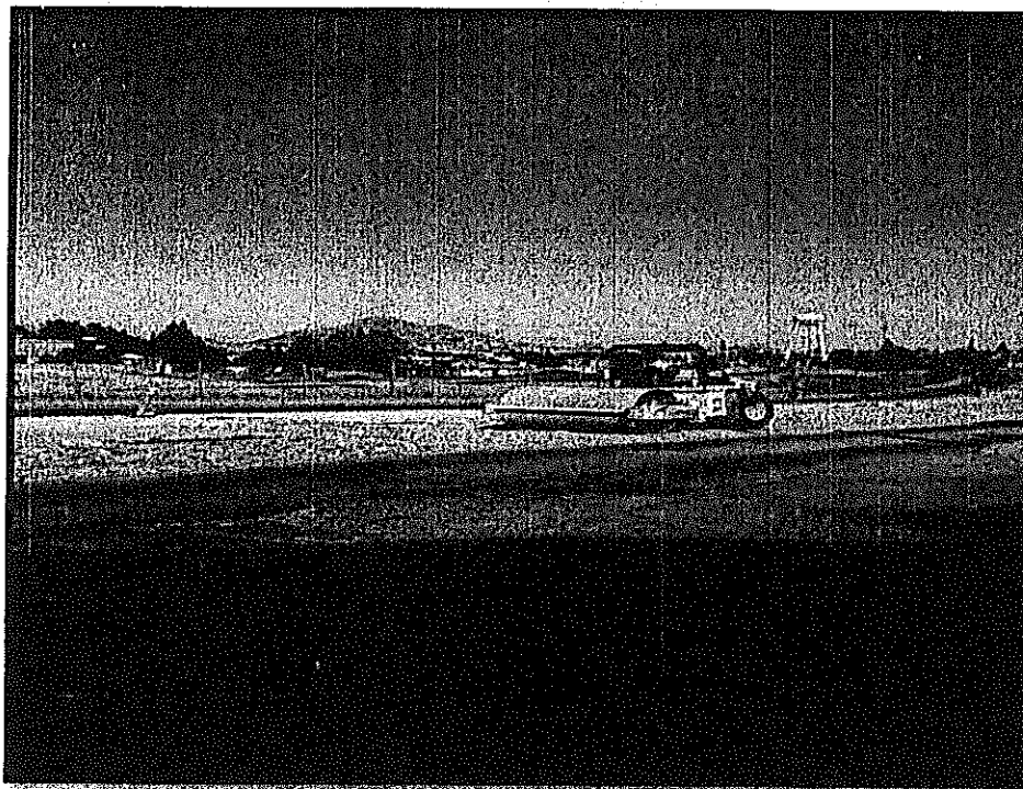
COMPACTADO DE FILTRO DE PIEDRA
