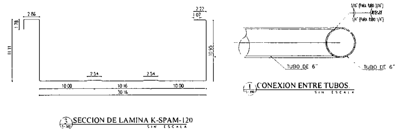
6-E DETALLES
