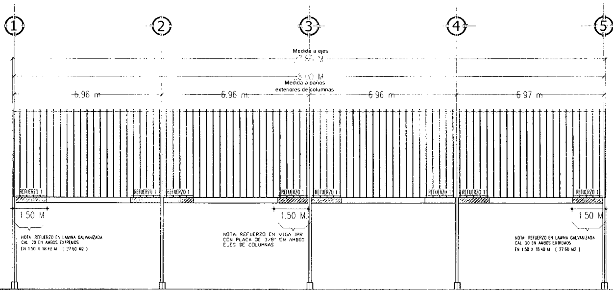
3-E CORTE ESTRUCTURAL LONGITUDINAL
