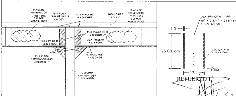
7-E DETALLES DE PLACAS DE CONEXION Y REFUERZO
