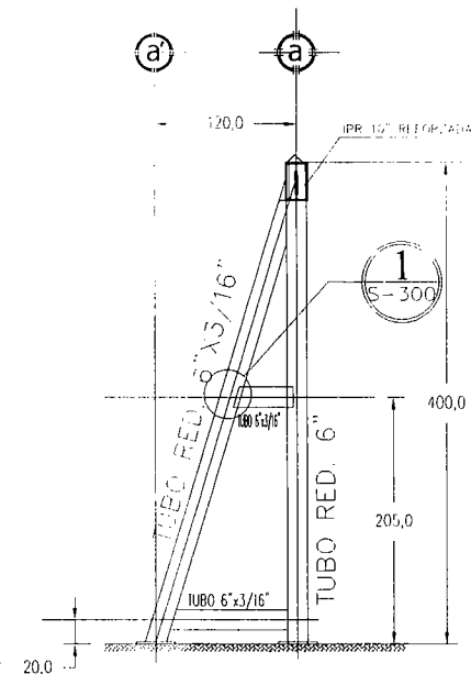
5-E SECCION DE COLUMNA
