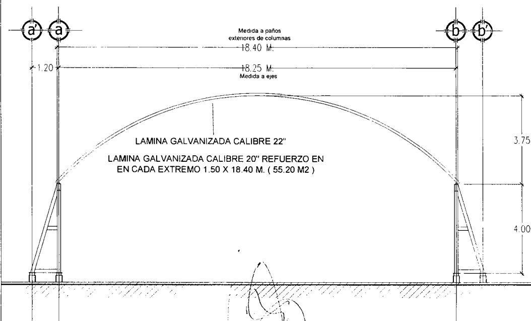
4-E CORTE TRANSVERSAL
