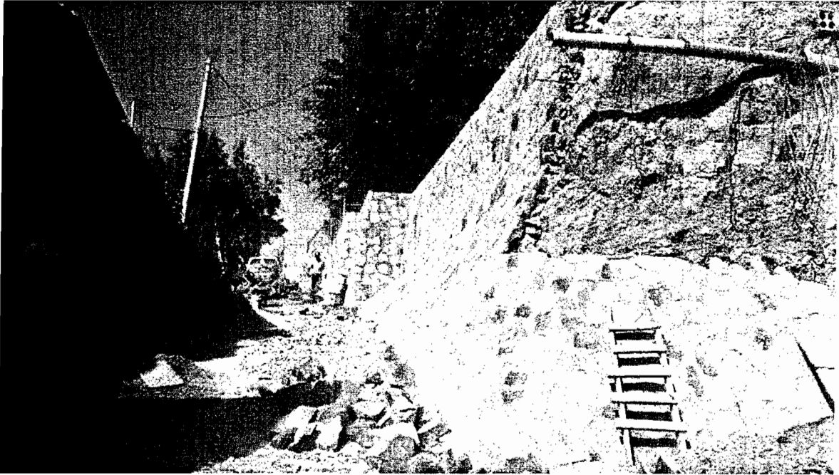
ZAMPEADO A BASE DE MAMPOSTERIA HASTA UNA ALTURA DE 6.10 M.
