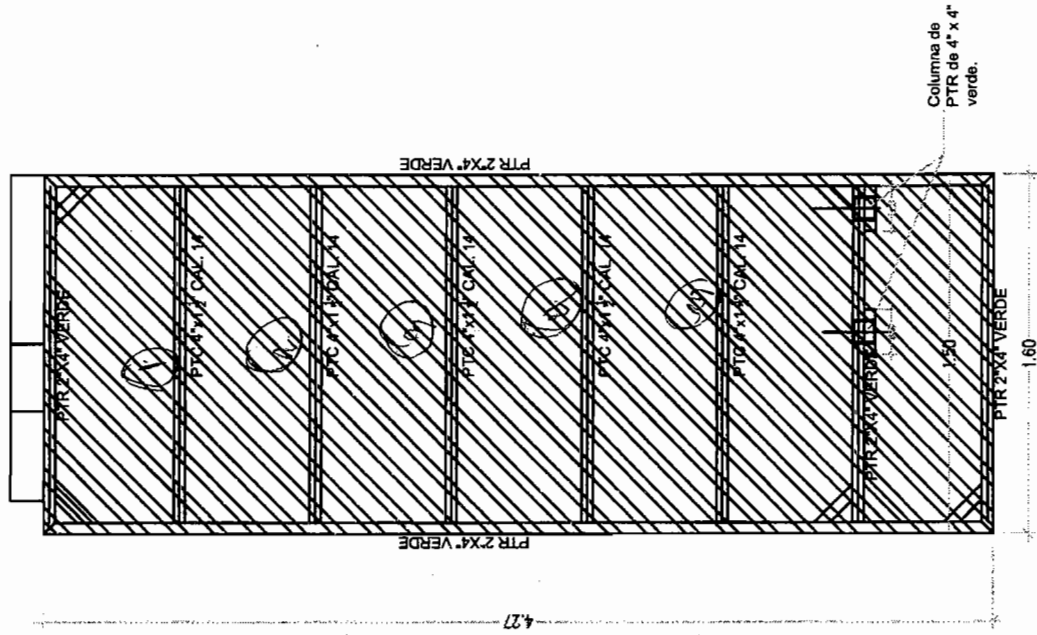
PLANTA ESTRUCTURAL
