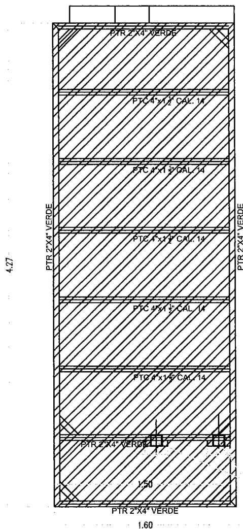
PLANTA ESTRUCTURAL
