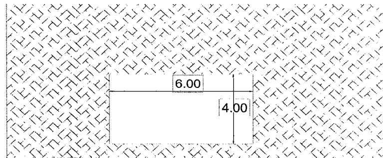
AREA DE ADOQUIN
