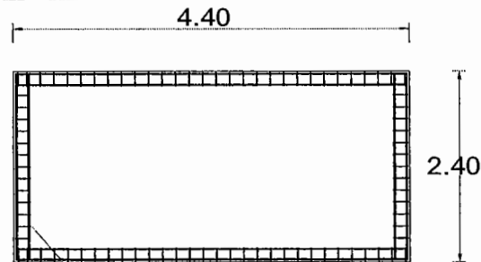
Trabe de Concreto armada con 4 varillas de 1/2" y estribos de 3/8" @ 15 cms.
