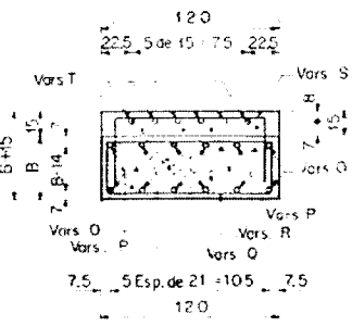
CORTE A-A
