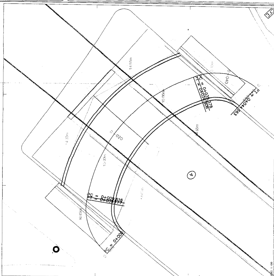
1 PLANTA GENERAL
