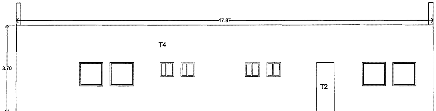
FACHADA TRASERA
