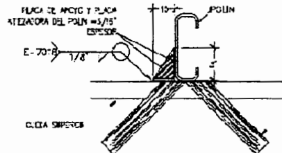
ELEVACION FRONTAL
