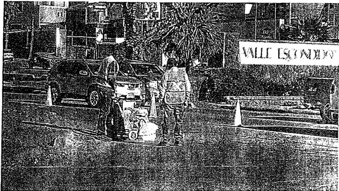
CORTE PARA CANALIZACION DEL CABLE
