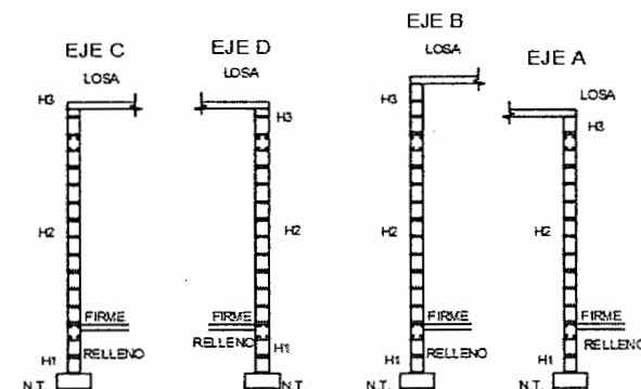
CORTES
