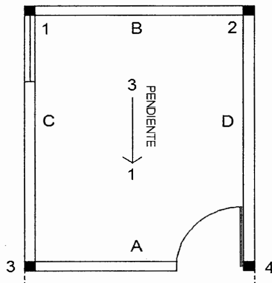
PLANTA
