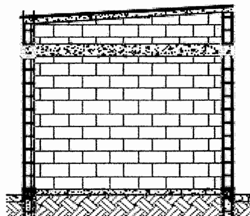
CORTES
