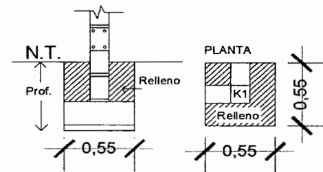
CIMENTACION
