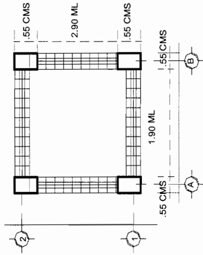
PLANTA ARQUITECTONICA
