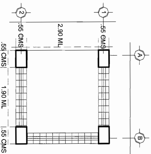
PLANTA ARQUITECTONICA
