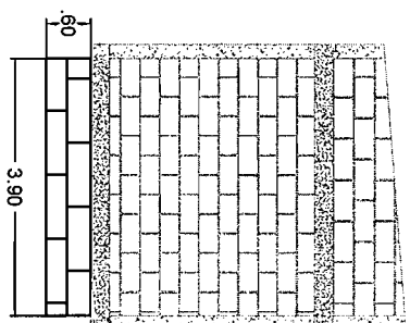
MURO 3
