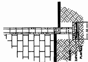
DETALLE CIMENTACION
