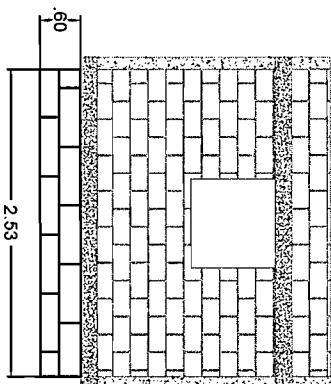
MURO 2
