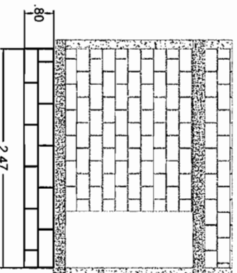
MURO 1
