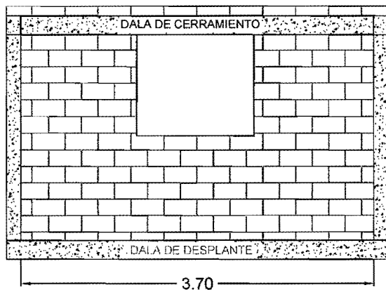
MURO 2
