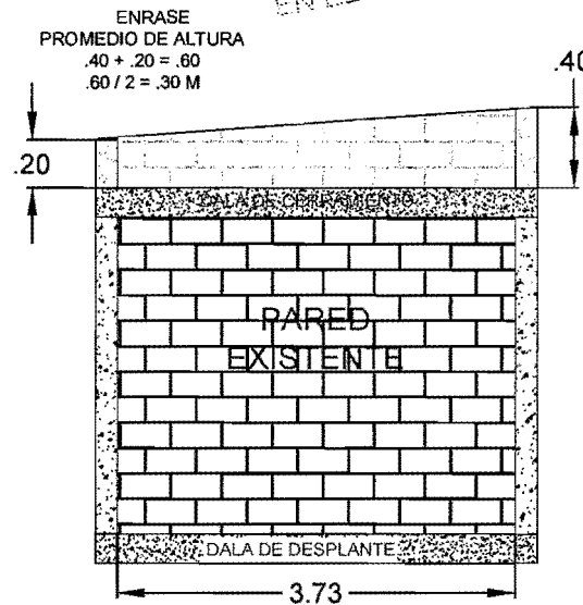
MURO 4
