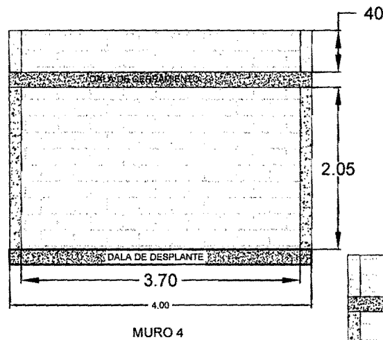
MURO 4
