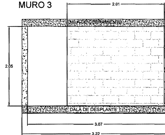
MURO 3
