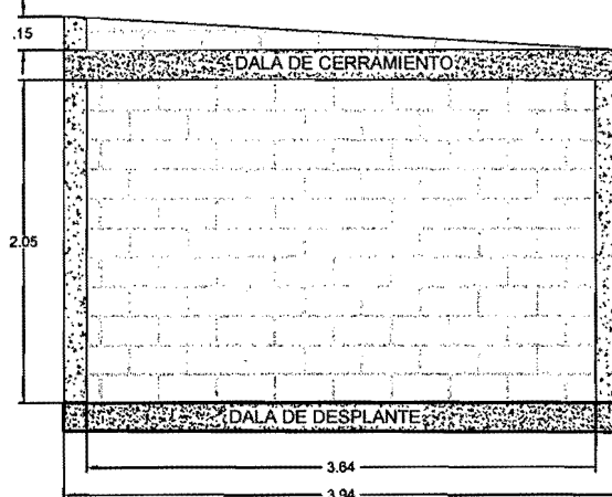
MURO 2
