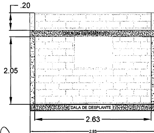
MURO 1
