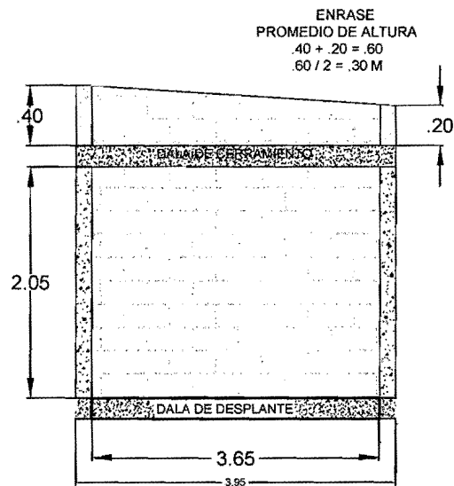
MURO 2
