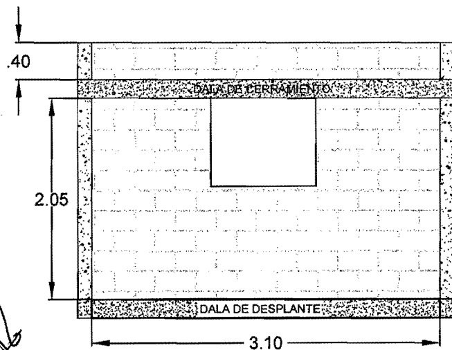
MURO 2
