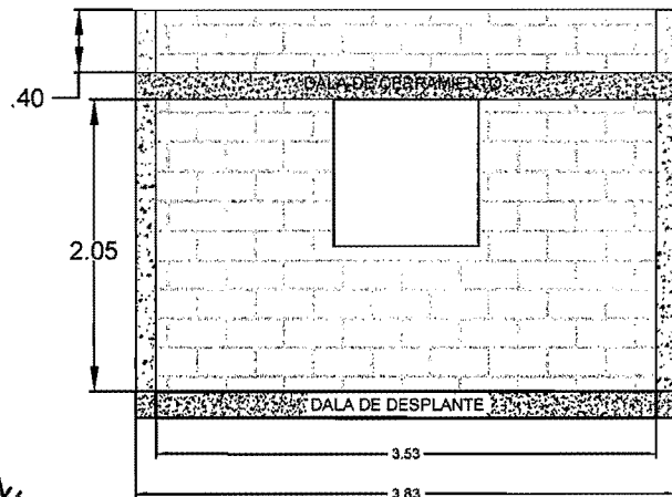
MURO 2
