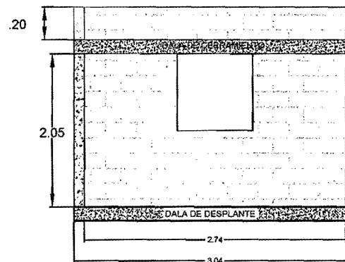
MURO 3
