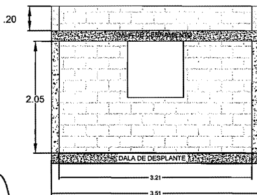
MURO 2
