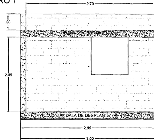
MURO 1
