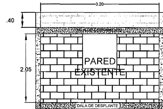
MURO 2
