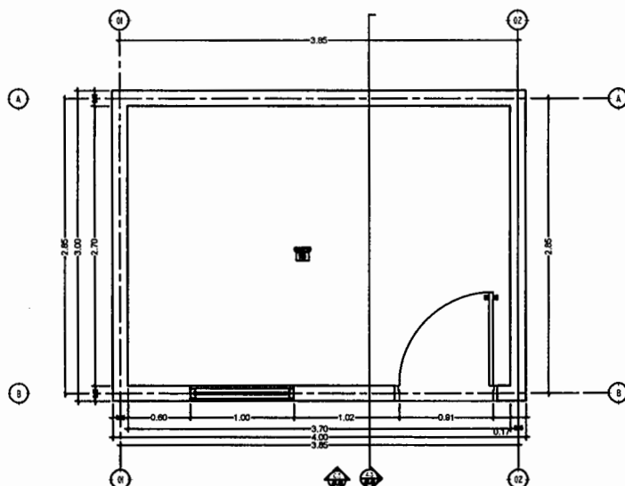
A6 PLANTA ARQUITECTONICA
