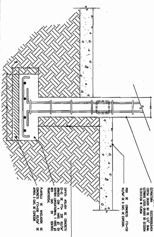
A3 DETALLE DE ZAPATA ANILADA (Z-A)
