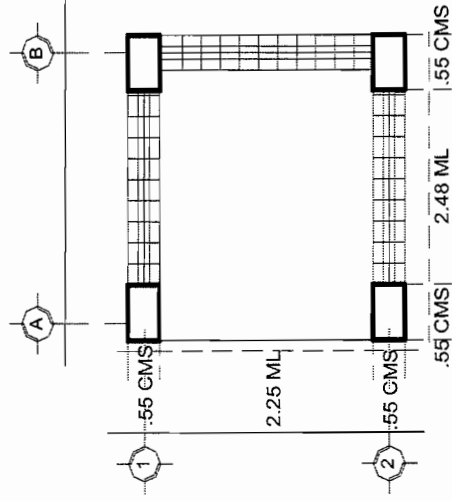
PLANTA ARQUITECTONICA
