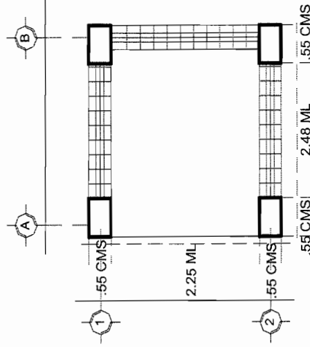
PLANTA ARQUITECTONICA
