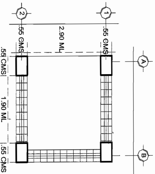
PLANTA ARQUITECTONICA
