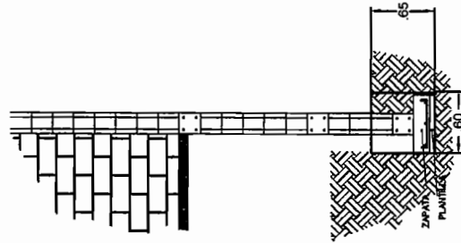
DETALLE DE EXCAVACION
