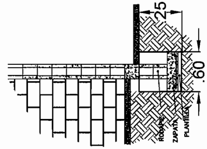
DETALLE DE EXCAVACION
