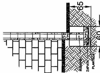
DETALLE DE EXCAVACIÓN
