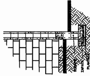
DETALLE DE UNIÓN
