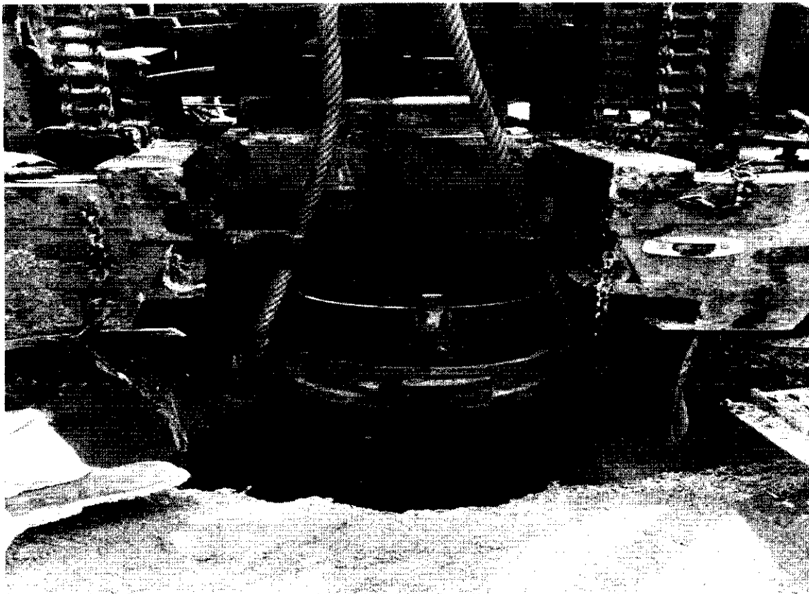
COLOCACION DE TUBERIA DE ADEME DE 14" DE DIAMETRO PARA CONTRA ADEME
