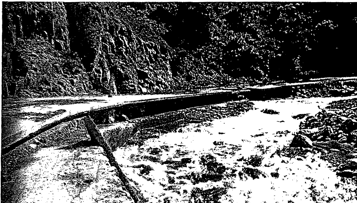
SOCAVACION EN EL TRAMO 21+830 AL 21+ 960
