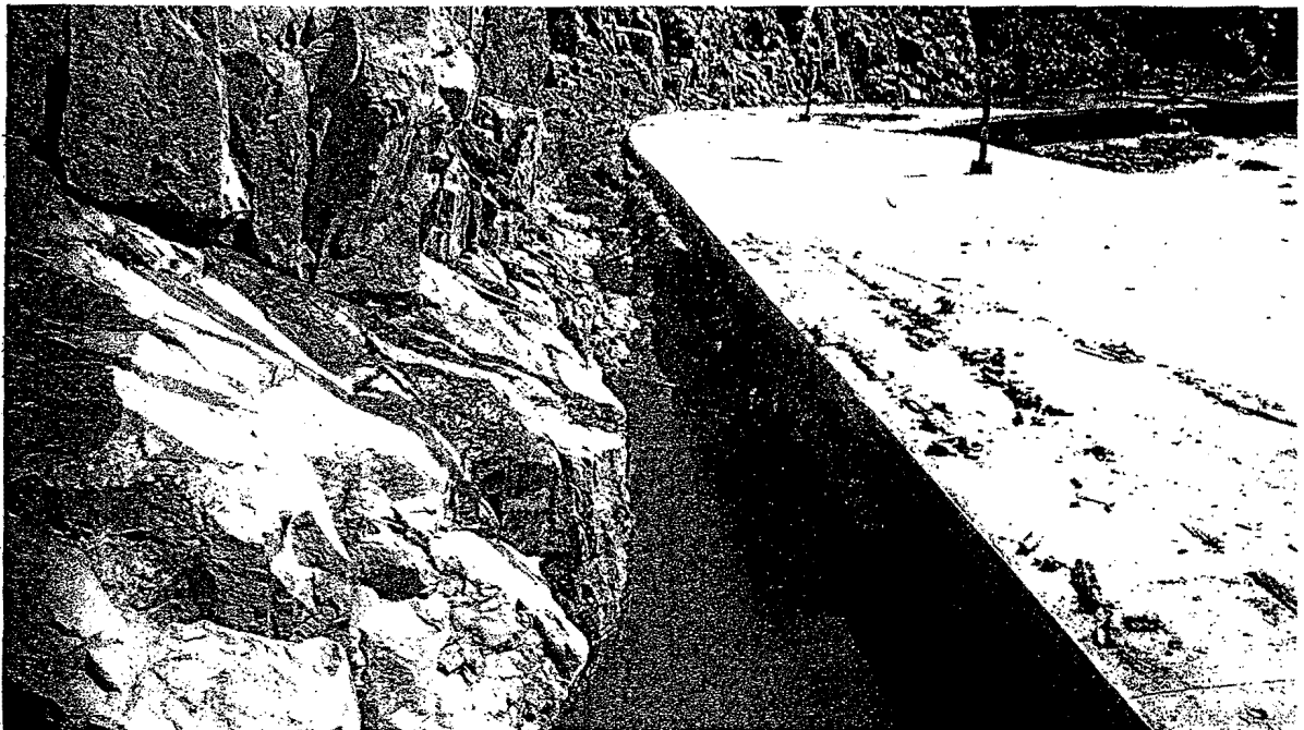
ARRASTRE DE MATERIAL EN EL AREA DE CUNETAS EN EL TRAMO 21+880 AL 21+960
