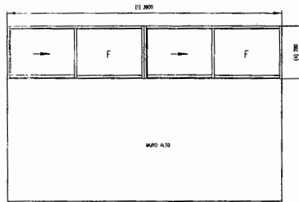
C2 ALZADO DE MURO ALTO EN AULAS
