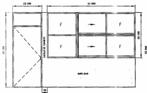
B1 ALZADO DE MURO BAJO EN AULAS
