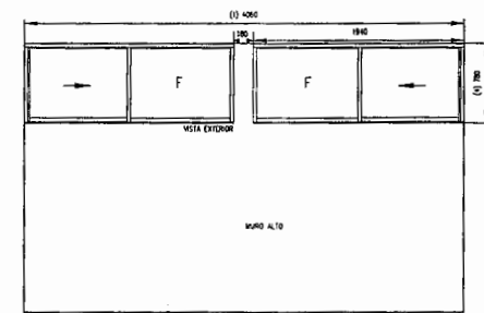
C2 ALZADO DE MURO ALTO EN SERVICIOS SANITARIOS
