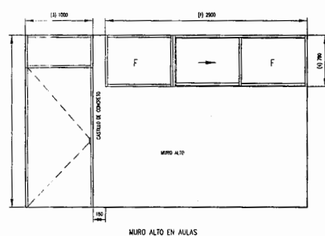
B2 ALZADO DE MURO ALTO EN AULAS
