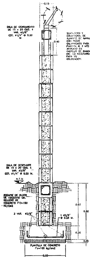
B1 DETALLE DE BARRA S/E
