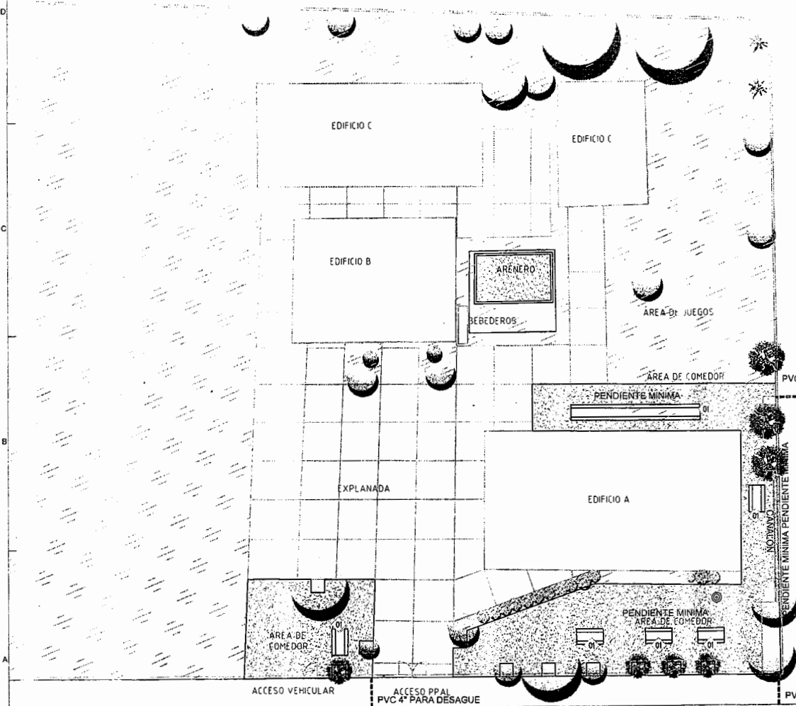
A6 PLANTA ARQUITECTÓNICA
