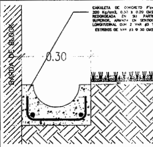
A1 DETALLE CANALON
