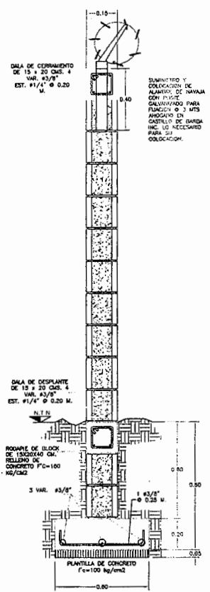
B1 DETALLE DE BARDA S/E
