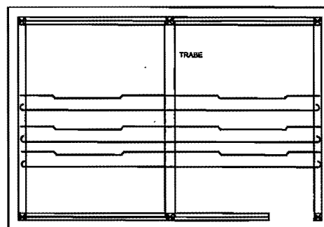
LOSA DE AZOTEA
