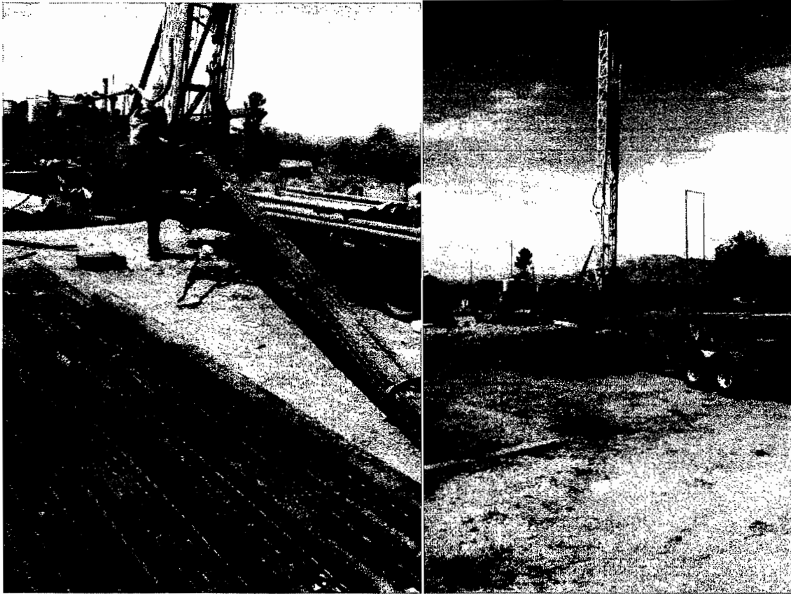
COLOCACION DE TUBERIA DE ADEME DE 8" DE DIAMETRO.
