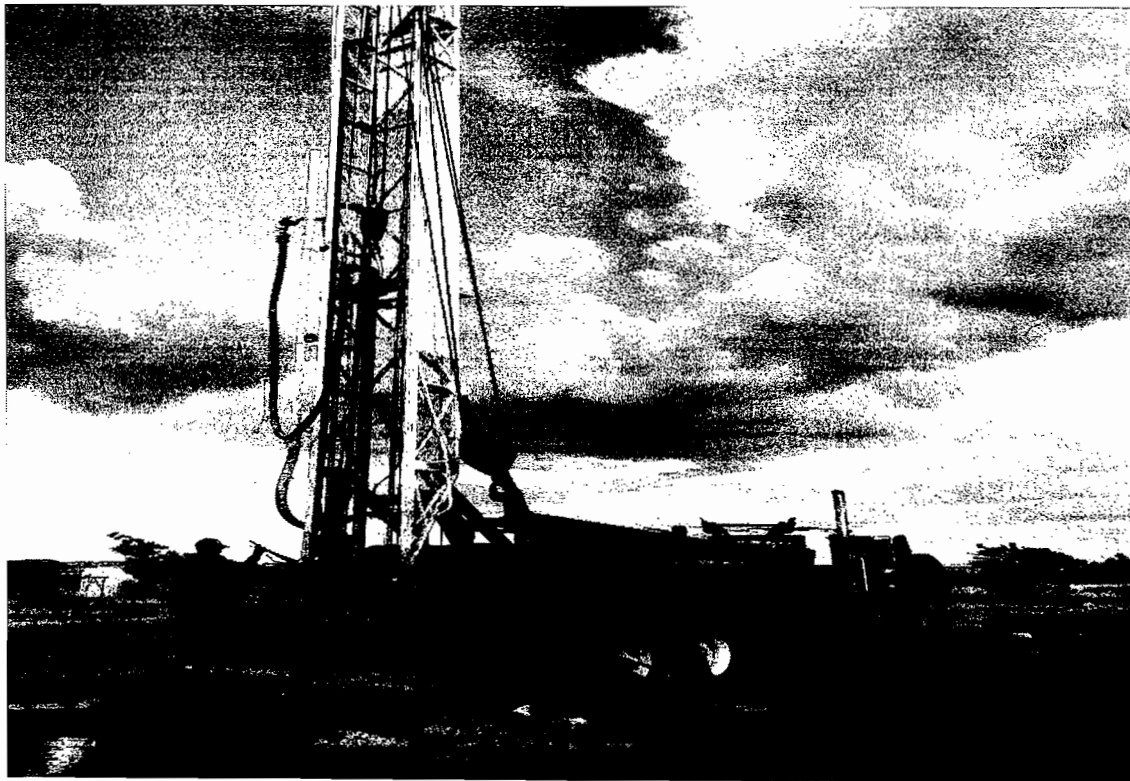
AMPLIACION DE AGUJERO DE 12" A 22" PARA ALOJAR TUBERIA DE CONTRADEME DE 14". 30 MTS.
