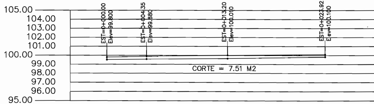
Perfil B-B' Cuadra 4
