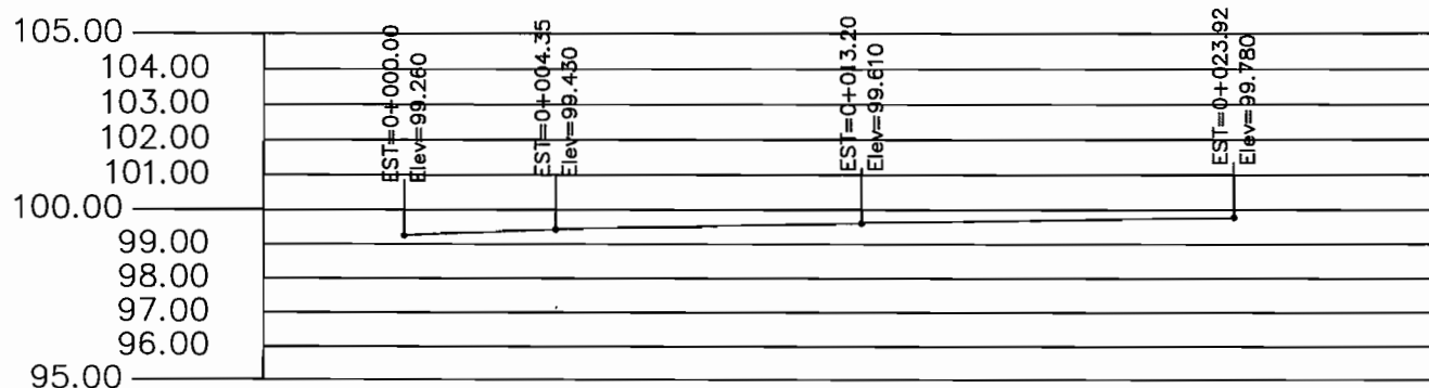
Perfil A-A' Cuadra 4
