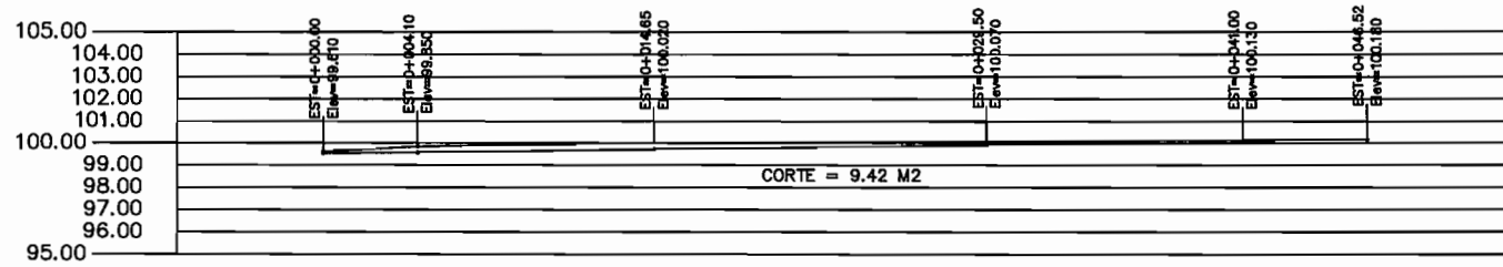
Perfil A-A' Cuadra 3
