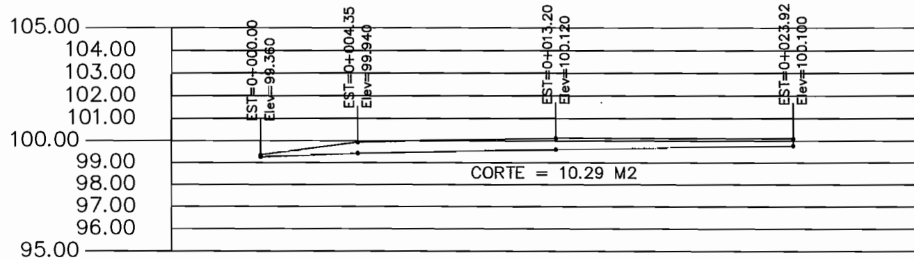
Perfil A-A' Cuadra 4
