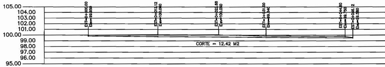
Perfil A-A' Cuadra 2
