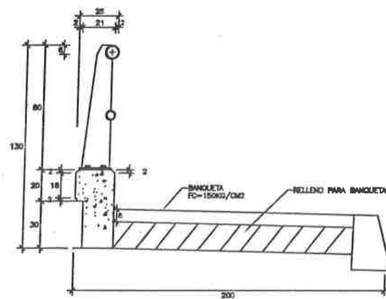
DETALLE DE BANQUETA (SOBRE PAVIMENTO)
