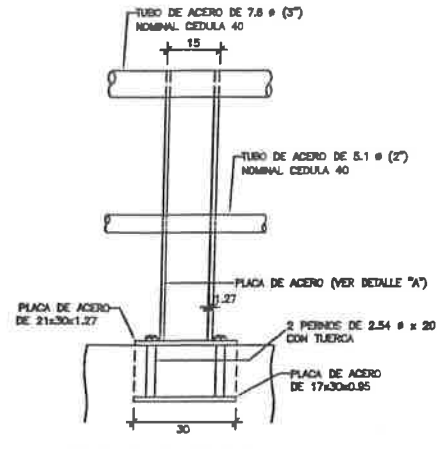
ELEVACION FRONTAL
