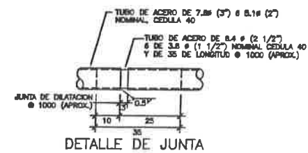
DETALLE DE JUNTA
