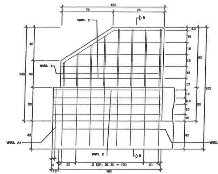
REMADE (EN PARAPETO)
