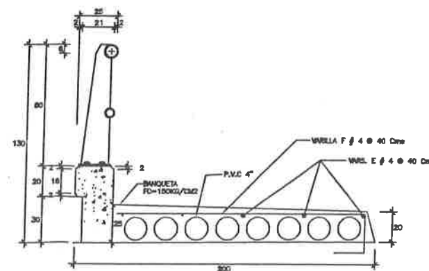
DETALLE DE BANQUETA (SOBRE LOSA)
