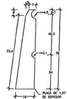
DETALLE "A"
