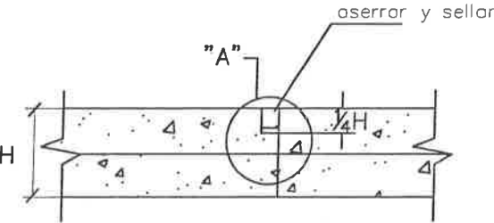
JUNTA TRANSVERSAL
