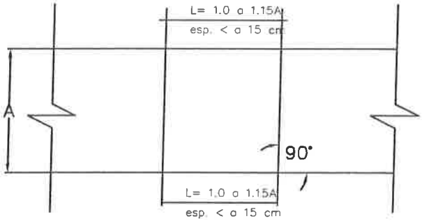
PROYECTO (LOSAS DE PAVIMENTO)
