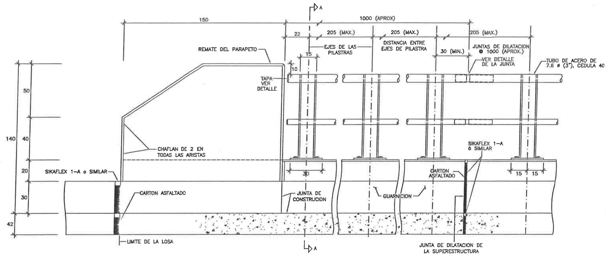
ELEVACION LATERAL
