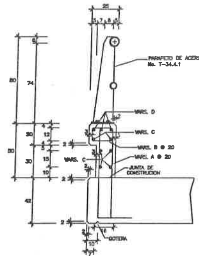
PARAPETO (SOBRE LOSA)
