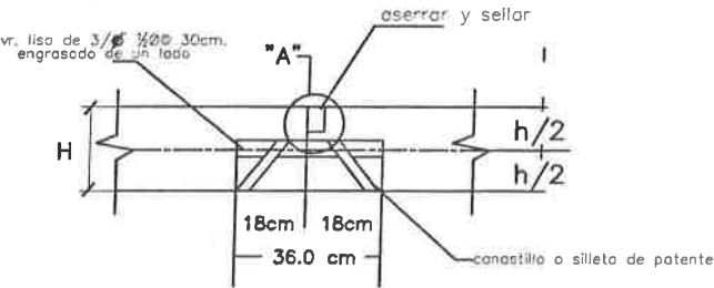
JUNTA TRANSVERSAL DE DILATACION
