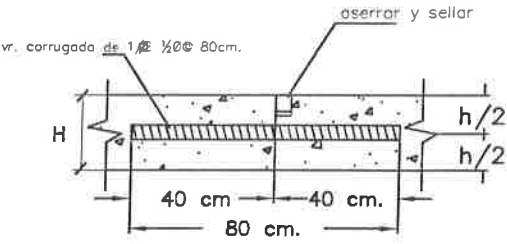
JUNTA LONGITUDINAL
