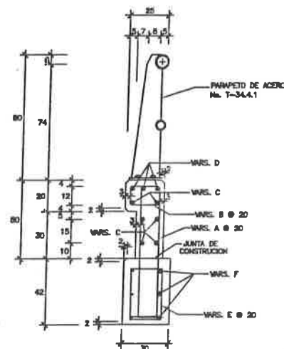
PARAPETO (SOBRE PAVIMENTO)
