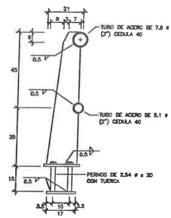
ELEVACION LATERAL
