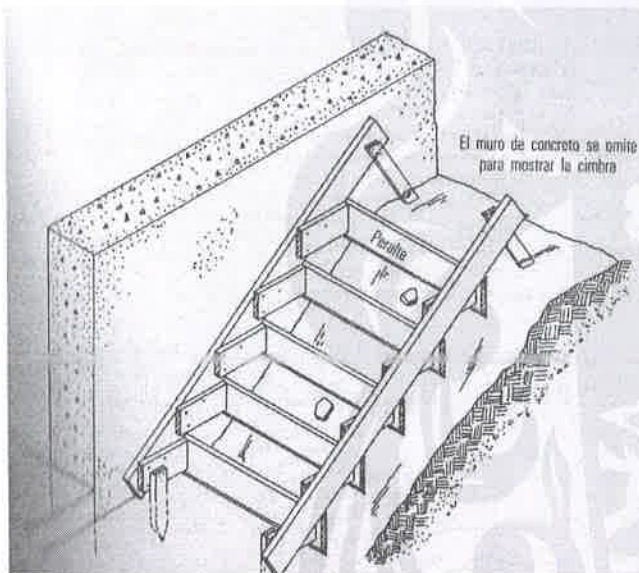
Detalle tipo para esta escalera
