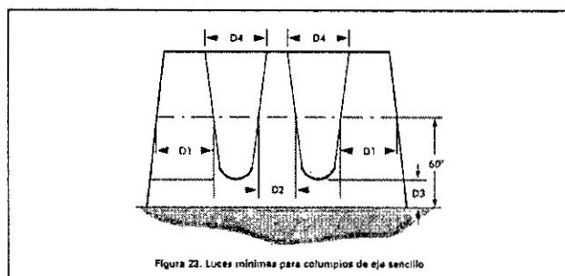
Figura 23. Luces mínimas para columpios de eje sencillo
